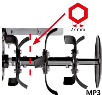
MP3 PRO
